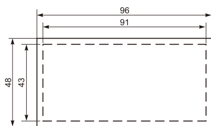
前视图
